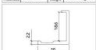
型号 FW-8512 名称 Model Name 壁厚 1.2mm 重量 0.186kg/m Thickness Weight
