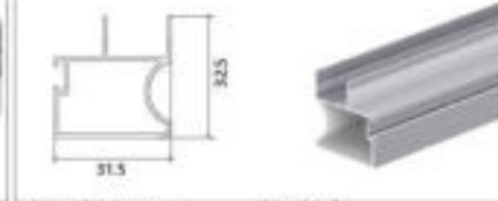
型号 Model CH-18 名称 Name 壁厚 Thickness 1.0mm 重量 Weight 0.36kg/m
