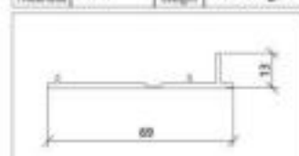
型号 FW-2004 名称 快装 Model Name Quick loading 壁厚 1.2mm 重量 0.428kg/m Thickness Weight
