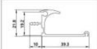
型号 AS-0265 名称 厚度 1.5mm 重量 0.413kg/m
