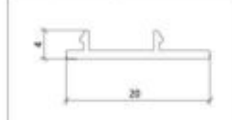
型号 FW-2006 名称 快装 Model Name Quick loading 壁厚 1.2mm 重量 0.08 kg/m Thickness Weight
