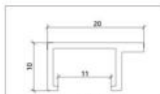
型号 FW-2007 名称 快装 Model Name Quick loading 壁厚 1.2mm 重量 0.138kg/m Thickness Weight
