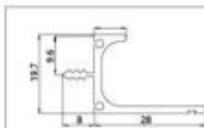
型号 XHH-004B 名称 厚度 mm 重量 0.292kg/m
