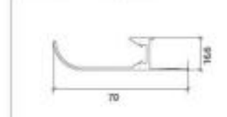
型号 FW-8472 名称 Model Name 壁厚 1.2mm 重量 0.408kg/m Thickness Weight
