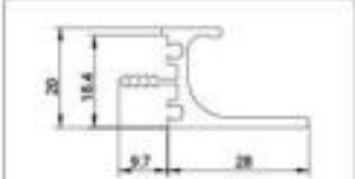
型号 AS-0266 名称 厚度 2.0mm 重量 0.389kg/m
