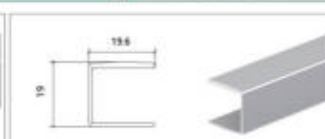
型号 Model KSW04 名称 Name 壁厚 Thickness 0.9mm 重量 Weight 0.175kg/m
