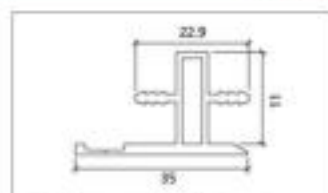
型号 FW-8527 名称 快装 Model Name Quick loading 壁厚 1.2mm 重量 0.35kg/m Thickness Weight
