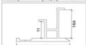
型号 FW-8513 名称 Model Name 壁厚 1.2mm 重量 0.33kg/m Thickness Weight
