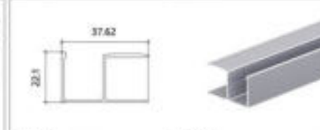
型号 Model KSW01A 名称 Name 壁厚 Thickness 1.0mm 重量 Weight 0.305kg/m
