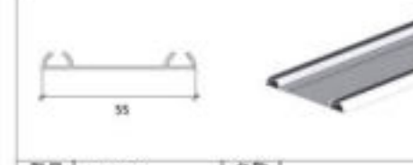
型号 Model KS308B 名称 Name 壁厚 Thickness mm 重量 Weight 0.183kg/m
