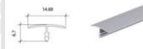
型号 Model XMNO.5 名称 Name 壁厚 Thickness 0.6mm 重量 Weight 0.041kg/m
