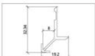
型号 FW-2003 名称 快装 Model Name Quick loading 壁厚 1.2mm 重量 0.217kg/m Thickness Weight
