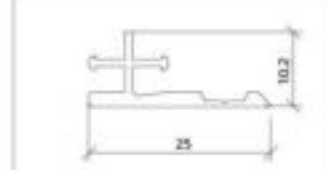
型号 FW-2009 名称 快装 Model Name Quick loading 壁厚 1.2mm 重量 0.161kg/m Thickness Weight
