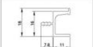
型号 AS-0287 名称 厚度 1.4mm 重量 0.196kg/m
