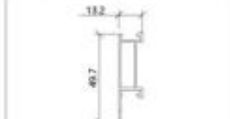
型号 FW-2008 名称 快装 Model Name Quick loading 壁厚 1.2mm 重量 0.335kg/m Thickness Weight
