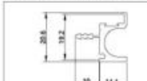
型号 AS-0268 名称 厚度 2.0mm 重量 0.251kg/m
