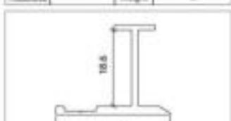
型号 FW-8517 名称 Model Name 壁厚 1.2mm 重量 0.244kg/m Thickness Weight
