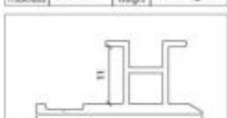
型号 FW-8524 名称 Model Name 壁厚 1.2mm 重量 0.305kg/m Thickness Weight
