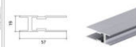
型号 Model 57x19 名称 Name 壁厚 Thickness mm 重量 Weight 0.766kg/m
