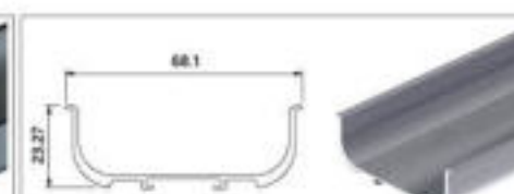
型号 FW-Q067 名称 拉手 厚度 1.8mm 重量 0.514kg/m
