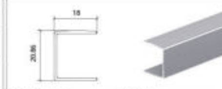
型号 Model KE04A 名称 Name 壁厚 Thickness 0.156mm 重量 Weight 1.0kg/m
