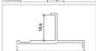
型号 FW-8516 名称 Model Name 壁厚 1.2mm 重量 0.336kg/m Thickness Weight
