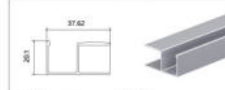
型号 Model KSW01 名称 Name 壁厚 Thickness 1.0mm 重量 Weight 0.293kg/m
