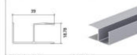
型号 Model KE01 名称 Name 壁厚 Thickness 0.9mm 重量 Weight 0.233kg/m
