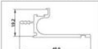
型号 AS-0269 名称 厚度 2.0mm 重量 0.398kg/m
