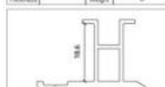
型号 FW-8515 名称 Model Name 壁厚 1.2mm 重量 0.355kg/m Thickness Weight
