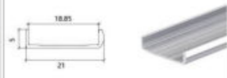
型号 Model CH-U21 名称 Name 壁厚 Thickness mm 重量 Weight 0.062kg/m
