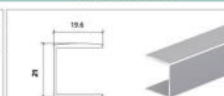
型号 Model KSW04A 名称 Name 壁厚 Thickness 0.9mm 重量 Weight 0.18kg/m
