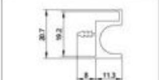
型号 AS-0165 名称 厚度 1.8mm 重量 0.273kg/m
