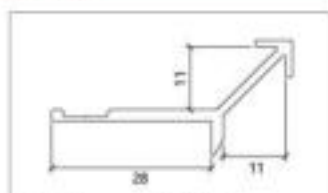
型号 FW-8528 名称 快装 Model Name Quick loading 壁厚 1.2mm 重量 0.268kg/m Thickness Weight
