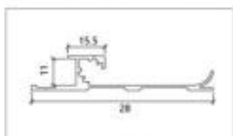
型号 FW-8529 名称 快装 Model Name Quick loading 壁厚 1.2mm 重量 0.464kg/m Thickness Weight
