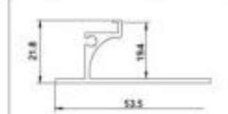
型号 AS-0159 名称 厚度 1.6mm 重量 0.404kg/m
