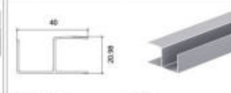
型号 Model KE01A 名称 Name 壁厚 Thickness 0.9mm 重量 Weight 0.242kg/m
