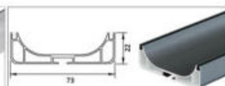
型号 SA-0369 名称 拉手 厚度 1.1mm 重量 0.667kg/m
