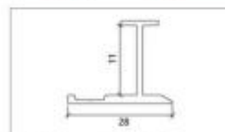
型号 FW-8526 名称 快装 Model Name Quick loading 壁厚 1.2mm 重量 0.213kg/m Thickness Weight
