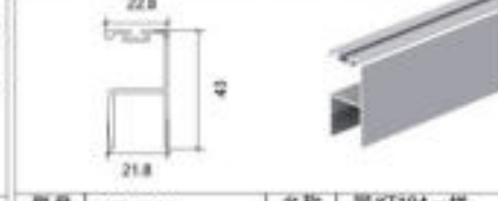
型号 Model KT194A 名称 Name 同KT194一样 壁厚 Thickness 1.1mm 重量 Weight 0.389kg/m
