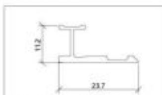
型号 FW-2001 名称 快装 Model Name Quick loading 壁厚 1.0mm 重量 0.155kg/m Thickness Weight
