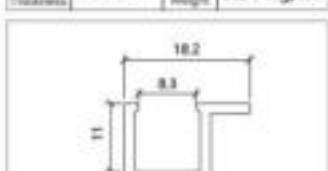
型号 FW-8521 名称 Model Name 壁厚 1.5mm 重量 0.168kg/m Thickness Weight
