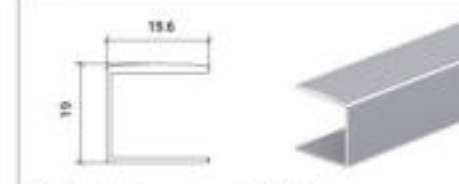
型号 Model KE04 名称 Name 壁厚 Thickness 0.9mm 重量 Weight 0.175kg/m
