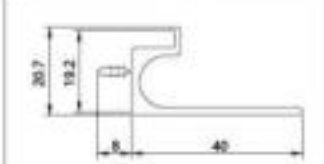
型号 AS-0164 名称 厚度 1.8mm 重量 0.413kg/m
