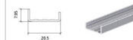
型号 Model DB-13 名称 Name 壁厚 Thickness mm 重量 Weight 0.089kg/m
