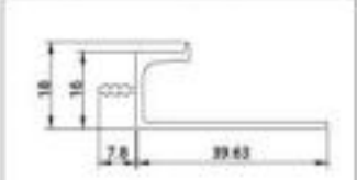
型号 AS-0288 名称 厚度 1.4mm 重量 0.305kg/m
