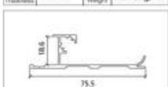
型号 FW-8520 名称 Model Name 壁厚 1.2mm 重量 0.486kg/m Thickness Weight
