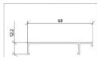
型号 FW-2005 名称 快装 Model Name Quick loading 壁厚 1.2mm 重量 0.311kg/m Thickness Weight
