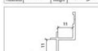
型号 FW-8523 名称 Model Name 壁厚 1.2mm 重量 0.355kg/m Thickness Weight
