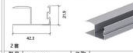
型号 Model XMNO.8 名称 Name 壁厚 Thickness 0.8mm 重量 Weight 0.301kg/m
